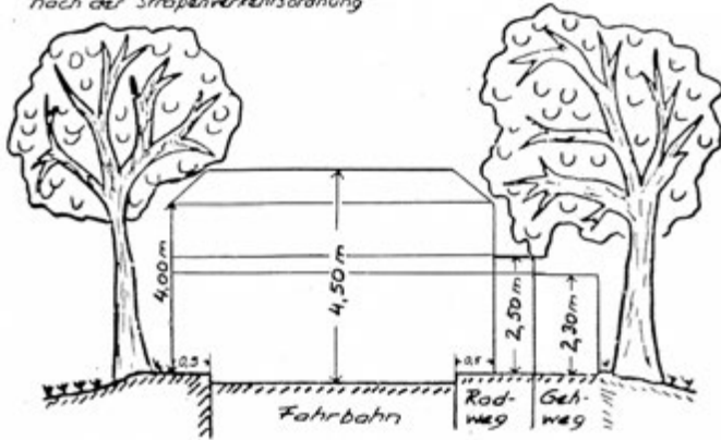
Lichtraumprofil nach der Straßenverkehrsordnung
